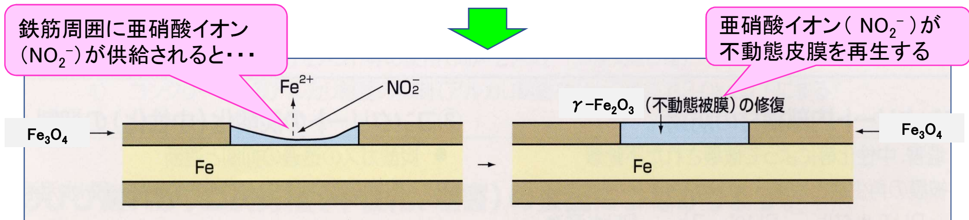
亜硝酸イオン( \text{NO}_2^- )による不動態被膜再生メカニズム
